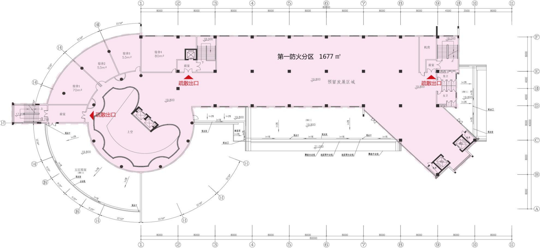
六层平面图 本层建筑面积 1677 平方米
