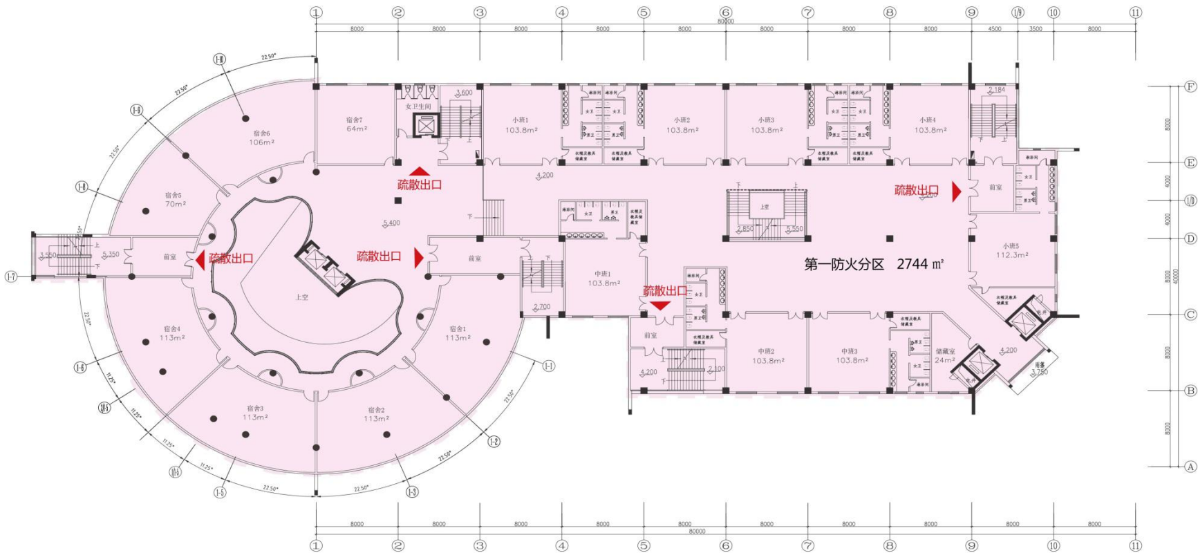
二层平面图
