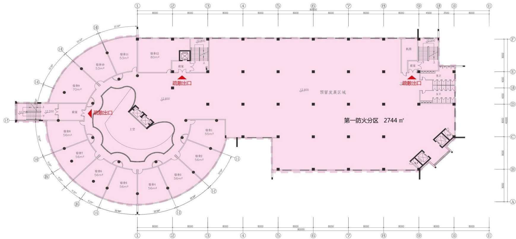
四层平面图
