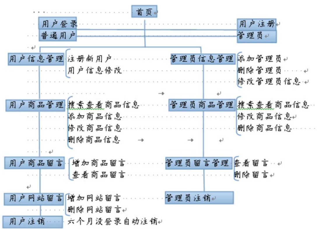
图 1 网站功能框架结构图
